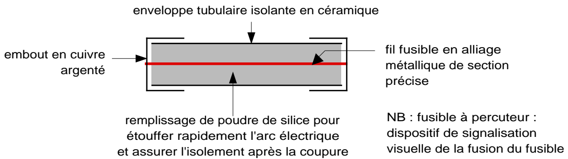
cartouche cylindrique
